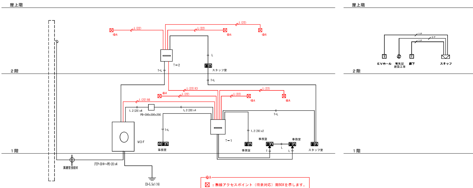
電話・情報設備 系統図
