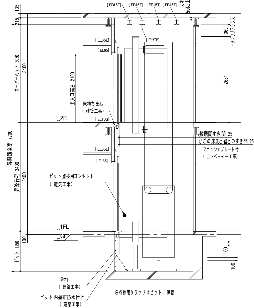
昇降路縦断面図
