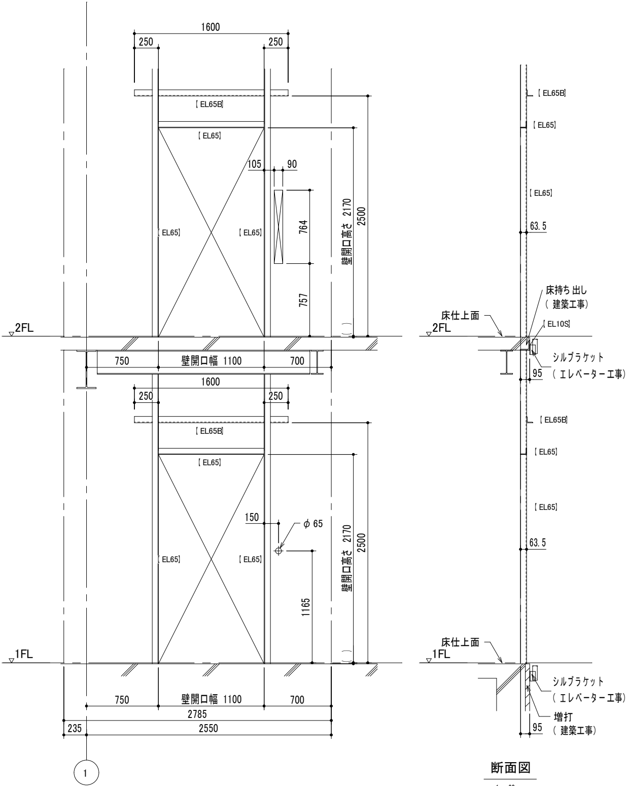
出入口壁穴明図
