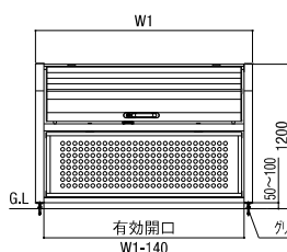
●寸法図(単位:mm) 単体
